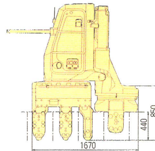
スーパーオート100
