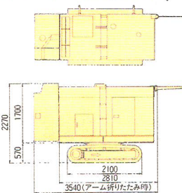
スーパーオート75油圧ユニット
