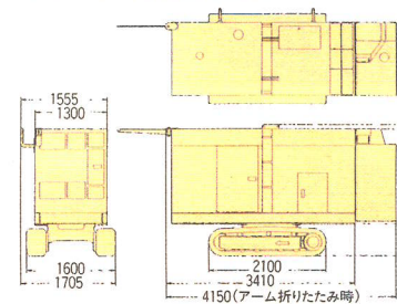
スーパーオート100油圧ユニット
